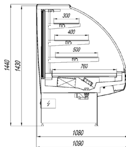
Рисунок 1. Внешний вид и сечение витрины ГРАНАТ 250
