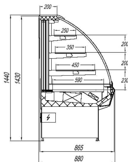
Рисунок 2. Внешний вид и сечение витрины ГРАНАТ КОМПАКТ 250
