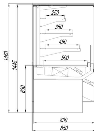
Рисунок 3. Внешний вид и сечение витрины ГРАНАТ КОМПАКТ КУБ 125
